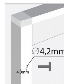
7. Nagwintować otwory gwintownikiem M5.
