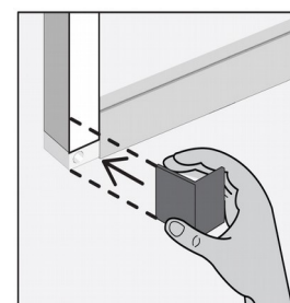
11. Założyć zaślepki narożników.
