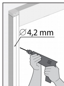
6. Przewiercić w połowie wysokości futrynę i stolarkę okienną.
