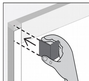
11. Założyć zaślepki narożników.
