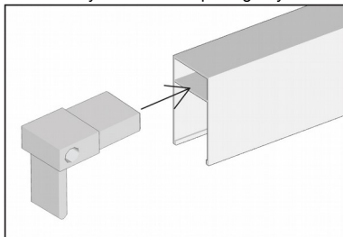
1. Założyć narożnik na profil górny.
