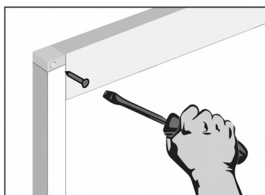
8. Wkręcić śrubę łączącą futrynę ze stolarką.
